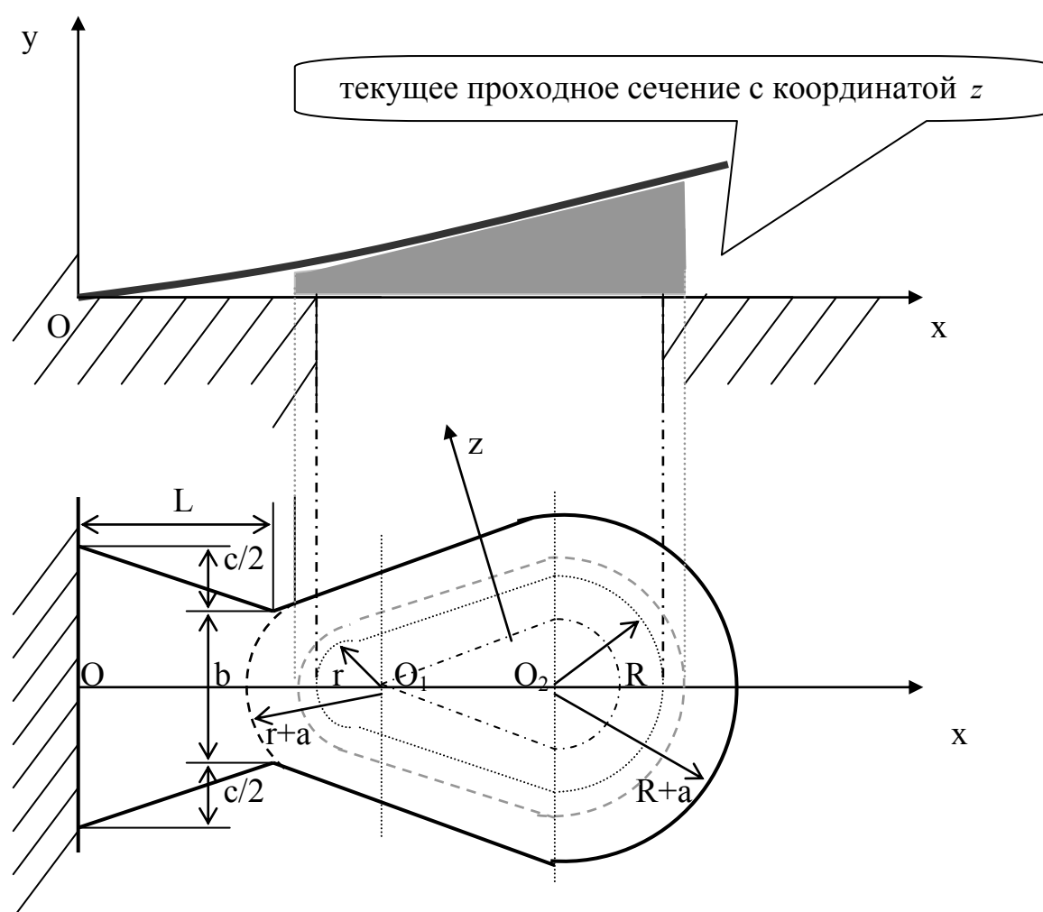
Рис. 1. Лепестковый клапан сложной геометрии.
