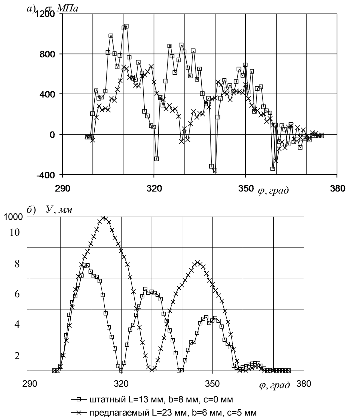
Рис. 2. Максимальные напряжения (а), возникающие в сечениях пластины, и перемещения конца пластины (б) для штатного и предлагаемого вариантов за цикл работы компрессора
