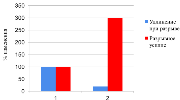
Рис. 1. Изменение механических характеристик желатиновых пленок, вызванных применением ТГ. 1- контрольный образец; 2- образец с ТГ
